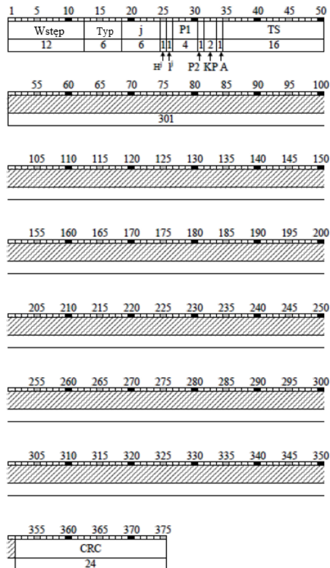
Rysunek B-7D. Nieprawidłowy ciąg danych L1OCd Typ 2
