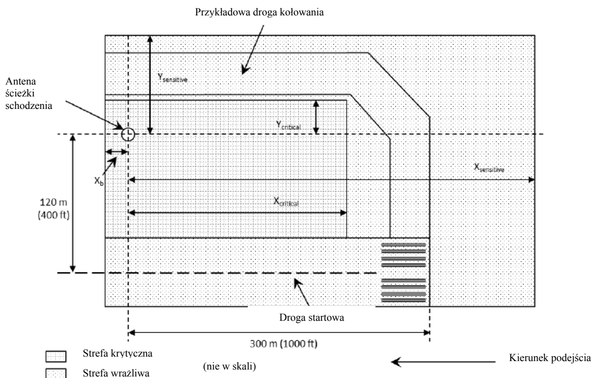
Rysunek C-4. Przykładowe wymiary strefy krytycznej i wrażliwej radiolaterny ścieżki schodzenia (wartości zawarte są w tabeli C-2A poniżej)
