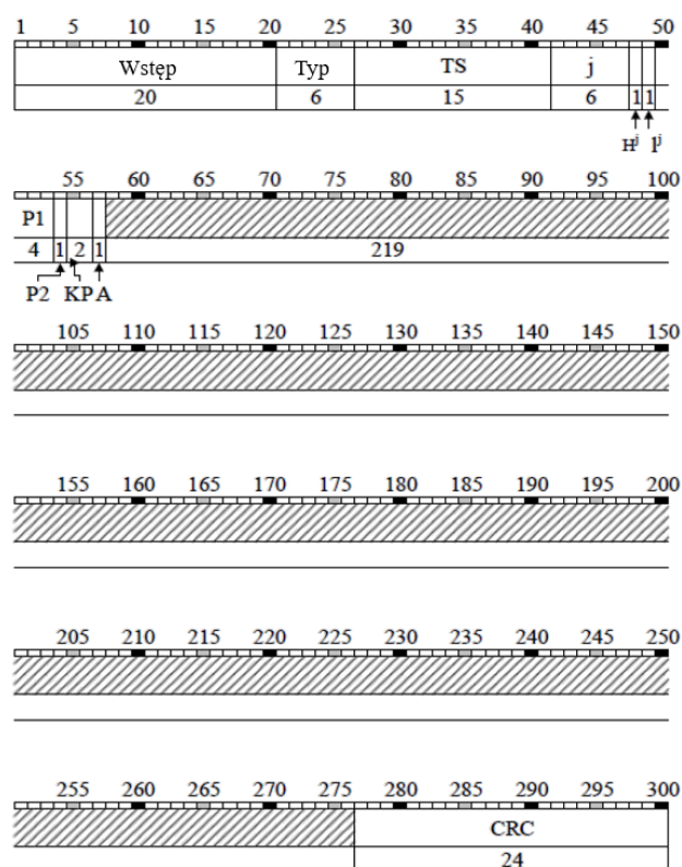
Rysunek B-8A. Ogólna struktura ciągu danych L3OCd
