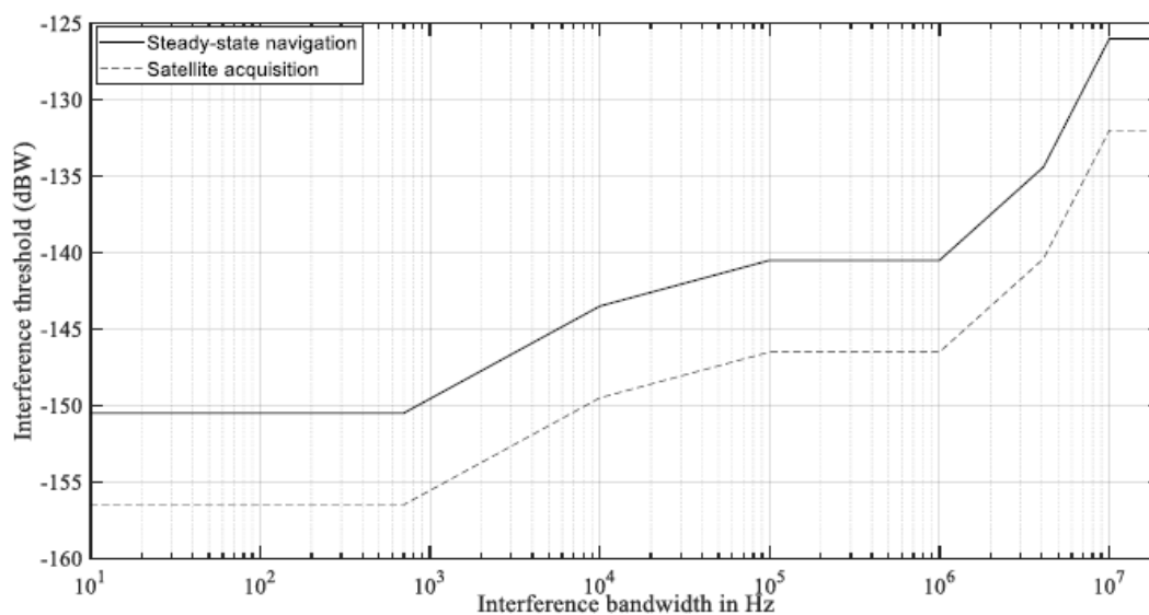
Rysunek RYS-08A. Progi zakłóceń a szerokość pasma dla odbiornika BDS B1I
