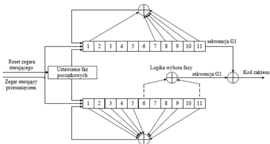
Rysunek B BDS-1. Generator CB1I
