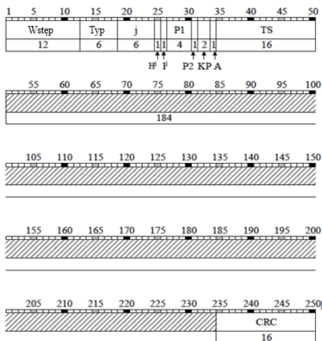
Rysunek B-7B. Ogólna struktura ciągu danych L1OCd
