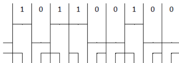
Rysunek D-19. Schemat kodowania bi-binarne (Manchester)
