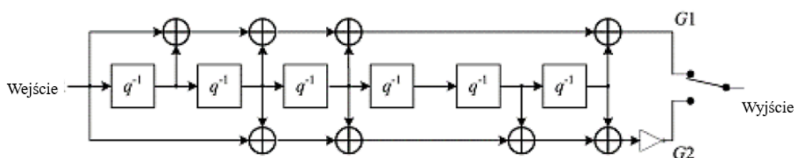
Rysunek GAL-4. Schemat kodowania konwolucyjnego F/NAV
