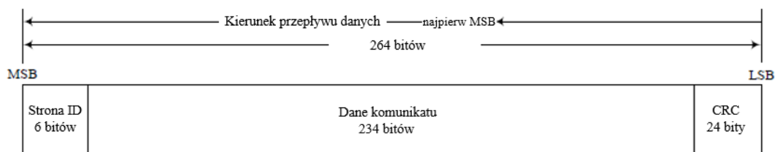
Rysunek B BDS-4. Struktura ramki dla podramki 3 B-CNAV1
